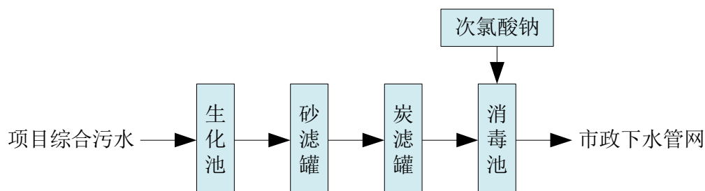
图 7-1 污水处理工艺流程图
